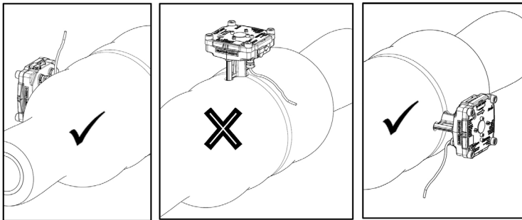
Obr.2: 130 ° -150 ° C s tepelnou izolací
