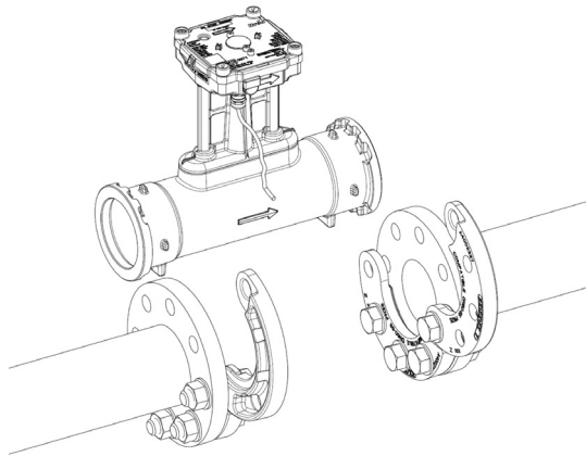
Abb.4: Installation mit Klappflanschen
