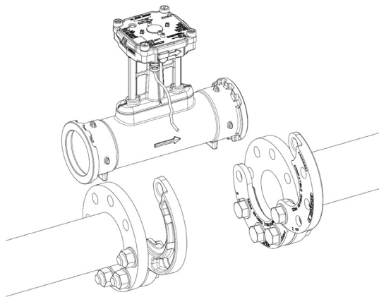
Fig N°4 : Installation AXONIC avec brides mobiles
