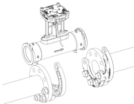
Rys. 4 Montaż przetwornika Axonic z ruchomymi kołnierzami.
