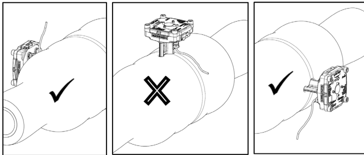
Fig N°2: 130°-150°C avec isolation thermique
