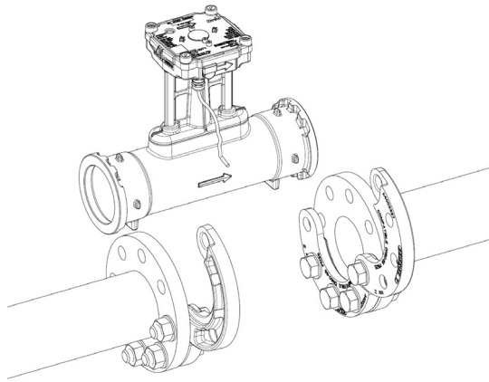
图4: 连接安装Axonic和专用活动法兰
