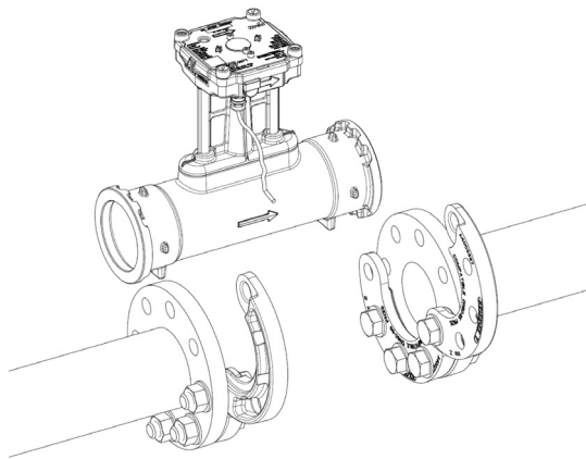
Slika 4: vgradnja merilnika pretoka AXONIC z mobilnima prirobnicama
