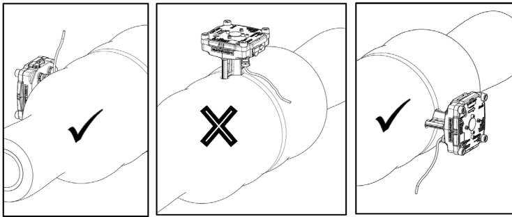
Рис. 2. Положение установки расходомера с теплоизоляцией при 130°- 150°C
