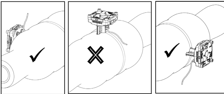
图2: 管道温度130° -150° C时, 积分仪正确安装位置
