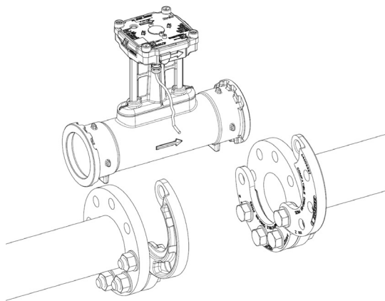
Fig. 4: installazione di AXONIC con flange mobili
