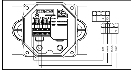
Collegamento AXONIC/C800
