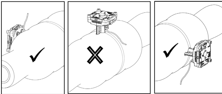
Slika 2: 130°-150°C s toplotno izolacijo
